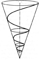
Figure 2. Une spirale logarithmique sur un cône.
